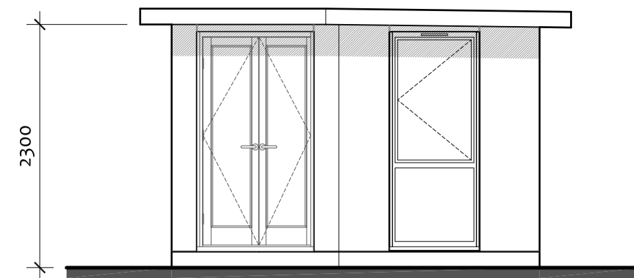
6 Side Elevation 3 Scale: 1:50
